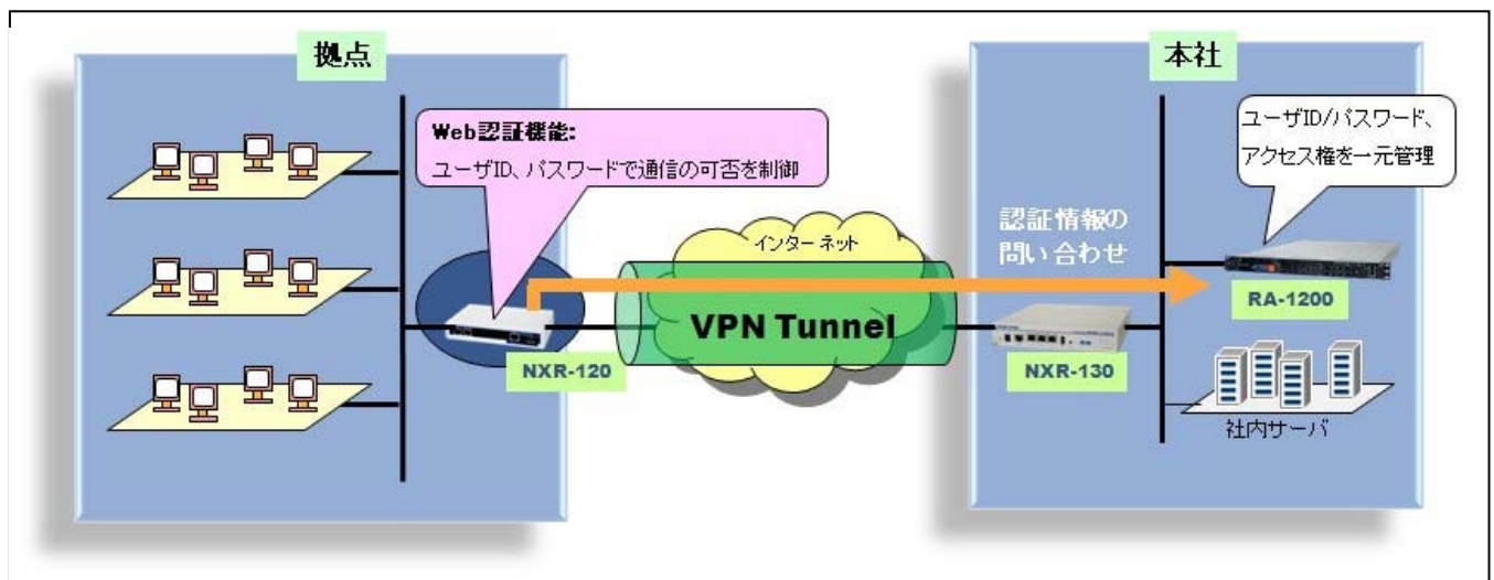
図 : FutureNet NXR シリーズ「Web 認証機能」と RA-1200 のソリューション
