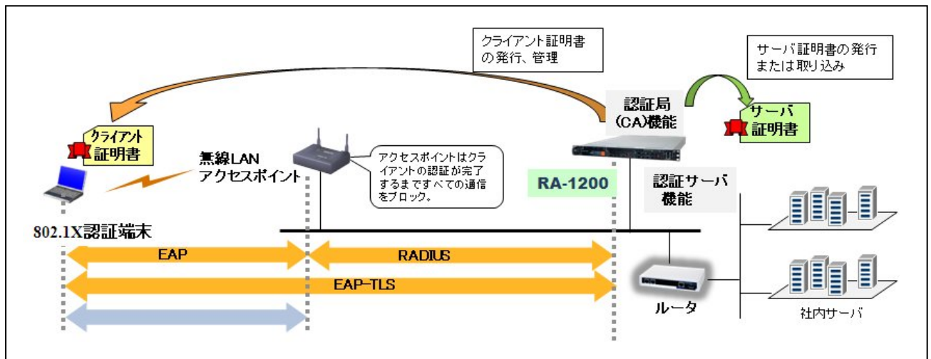
図: FutureNet RA-1200 による EAP-TLS 接続例
