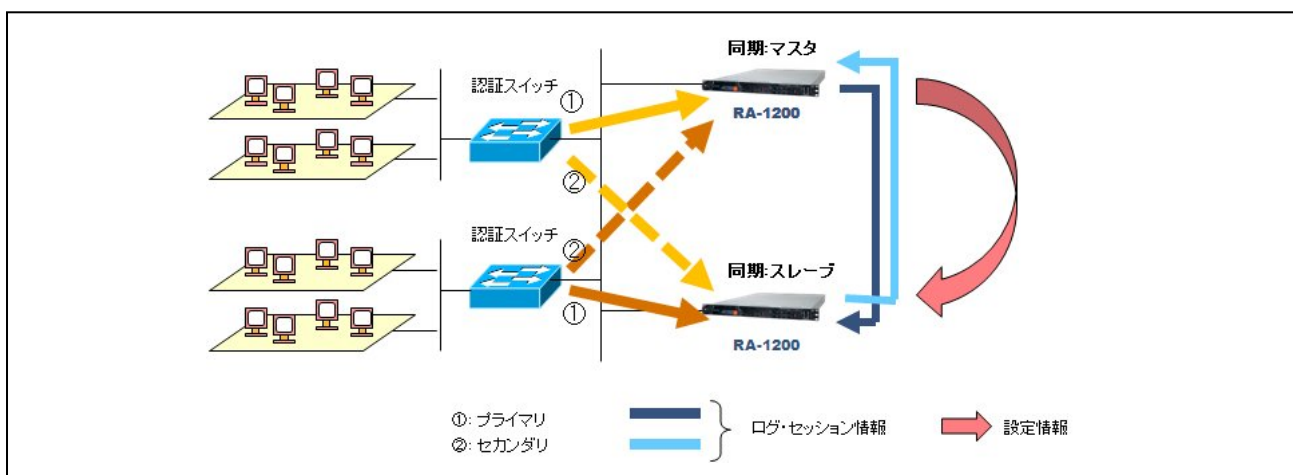
図: RA-1200 の Active-Active 方式による認証の冗長化と設定情報の同期
