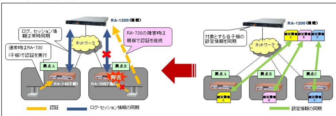
図: RA-1200 の親子連携機能による冗長化
