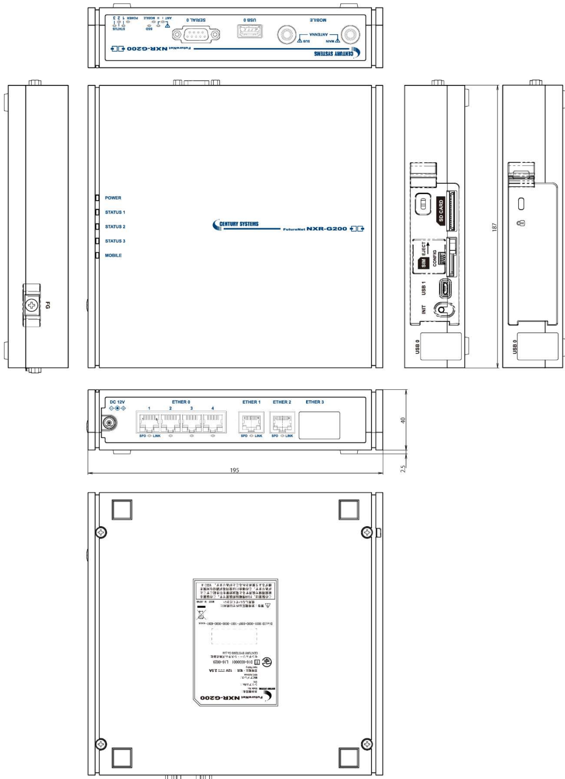
NXR-G240/L 外觀圖
