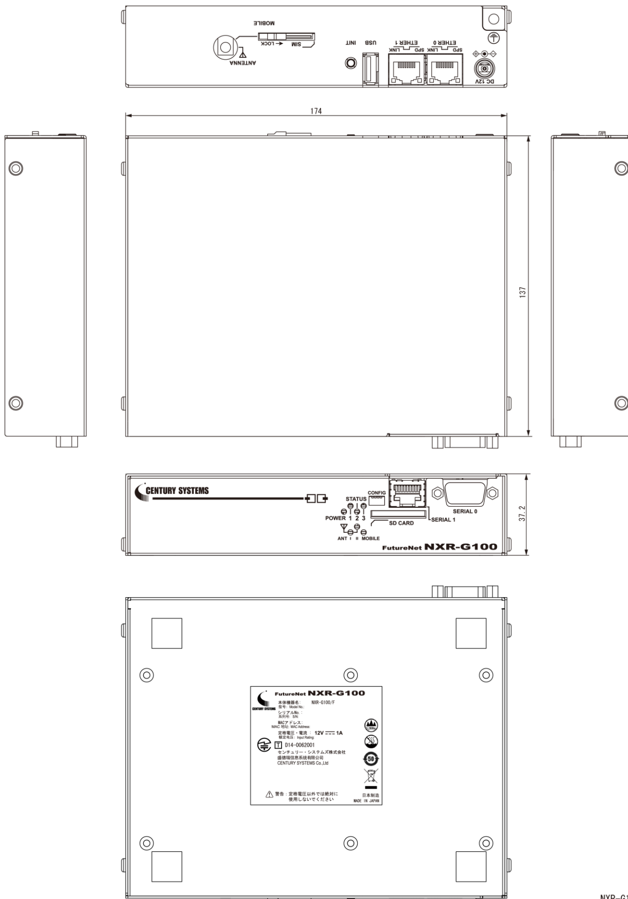
外觀図
