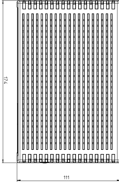
上面圖
