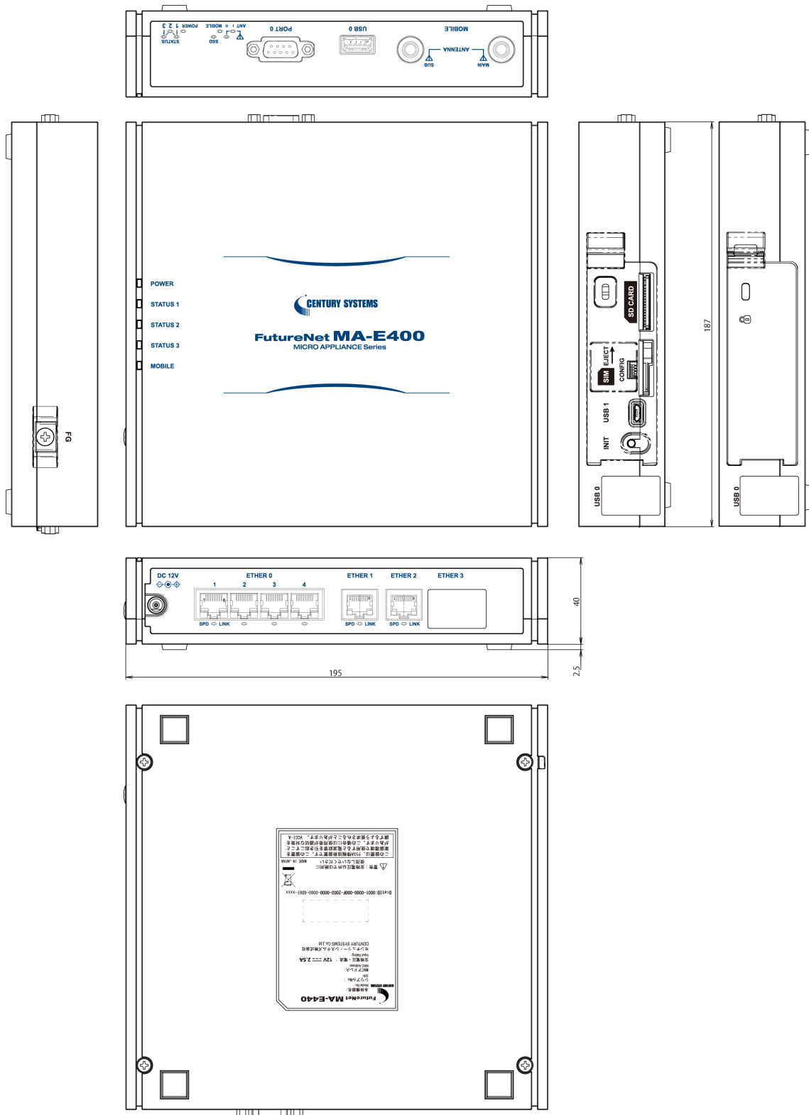
MA-E440/L 外觀圖
