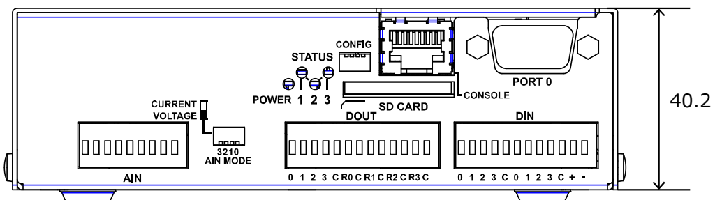
外觀圖
