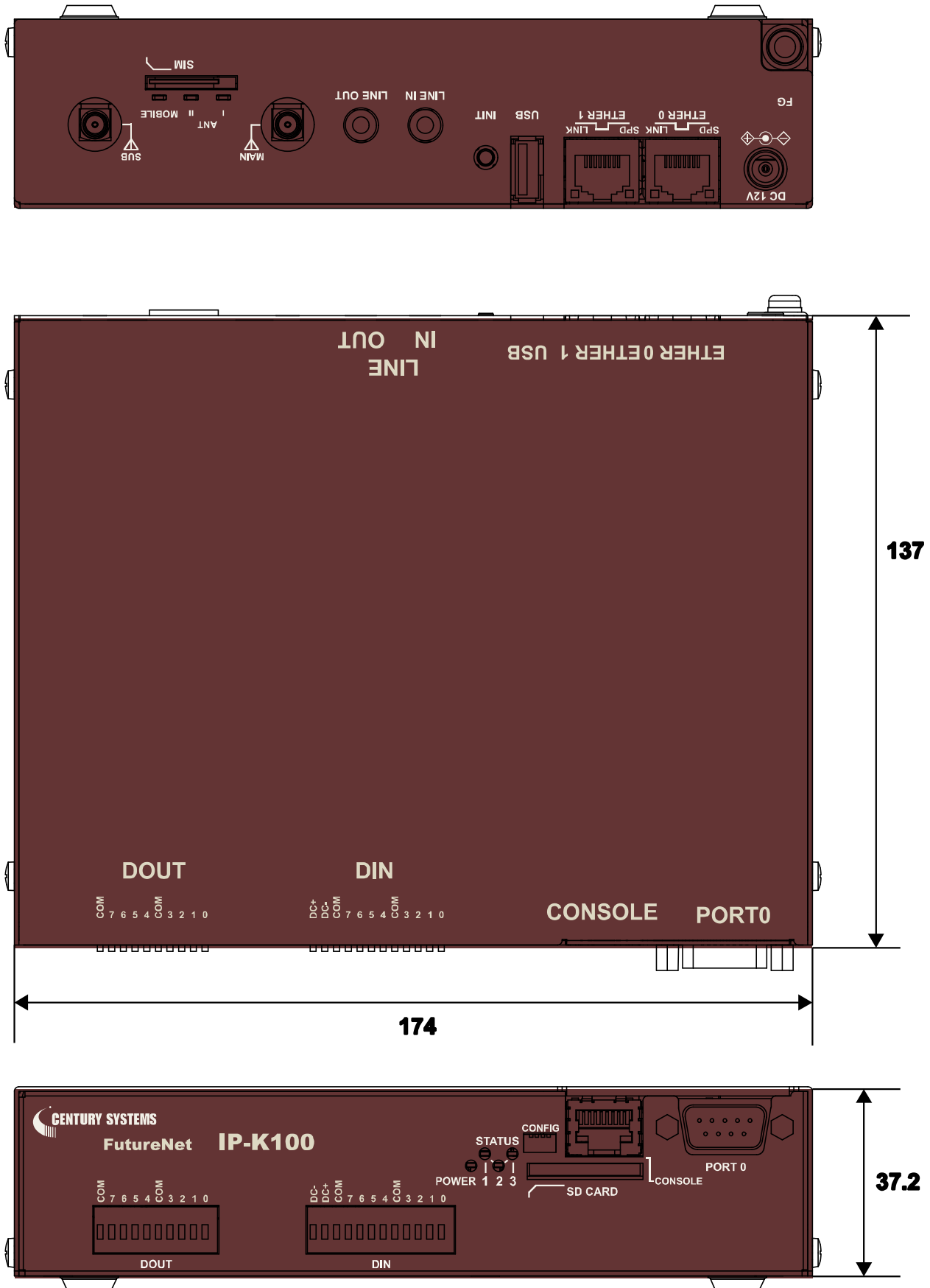
图 1 製品外觀図
