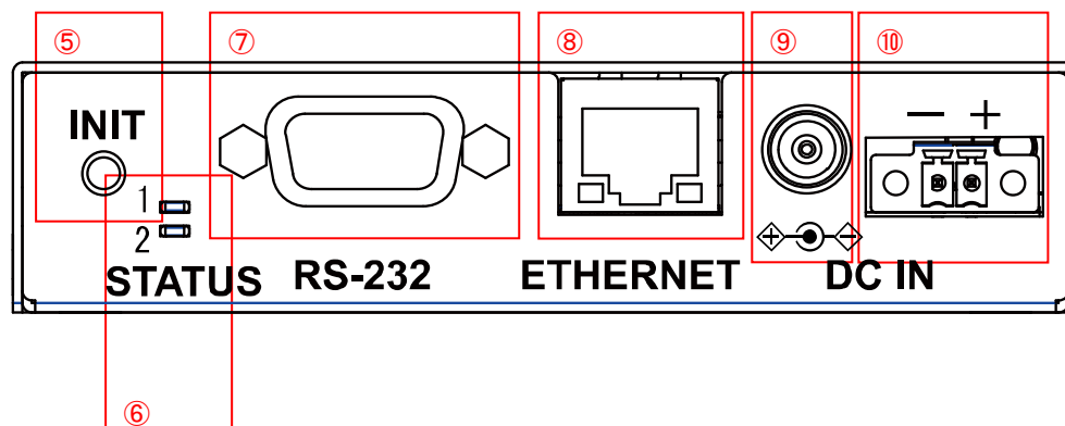
図 2 装置背面図
