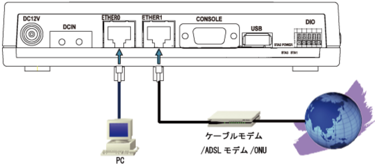
接続図 <例>
