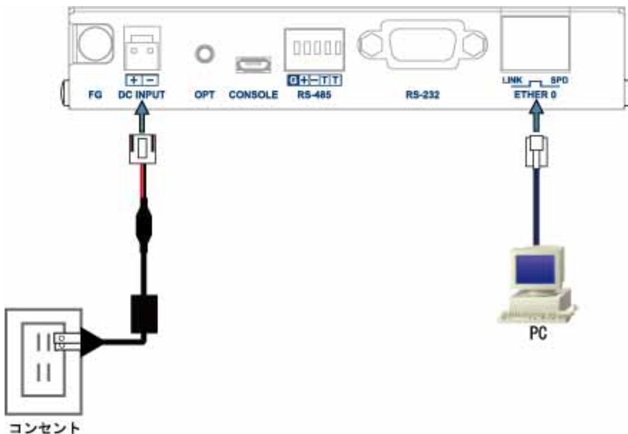
接続図<例>
