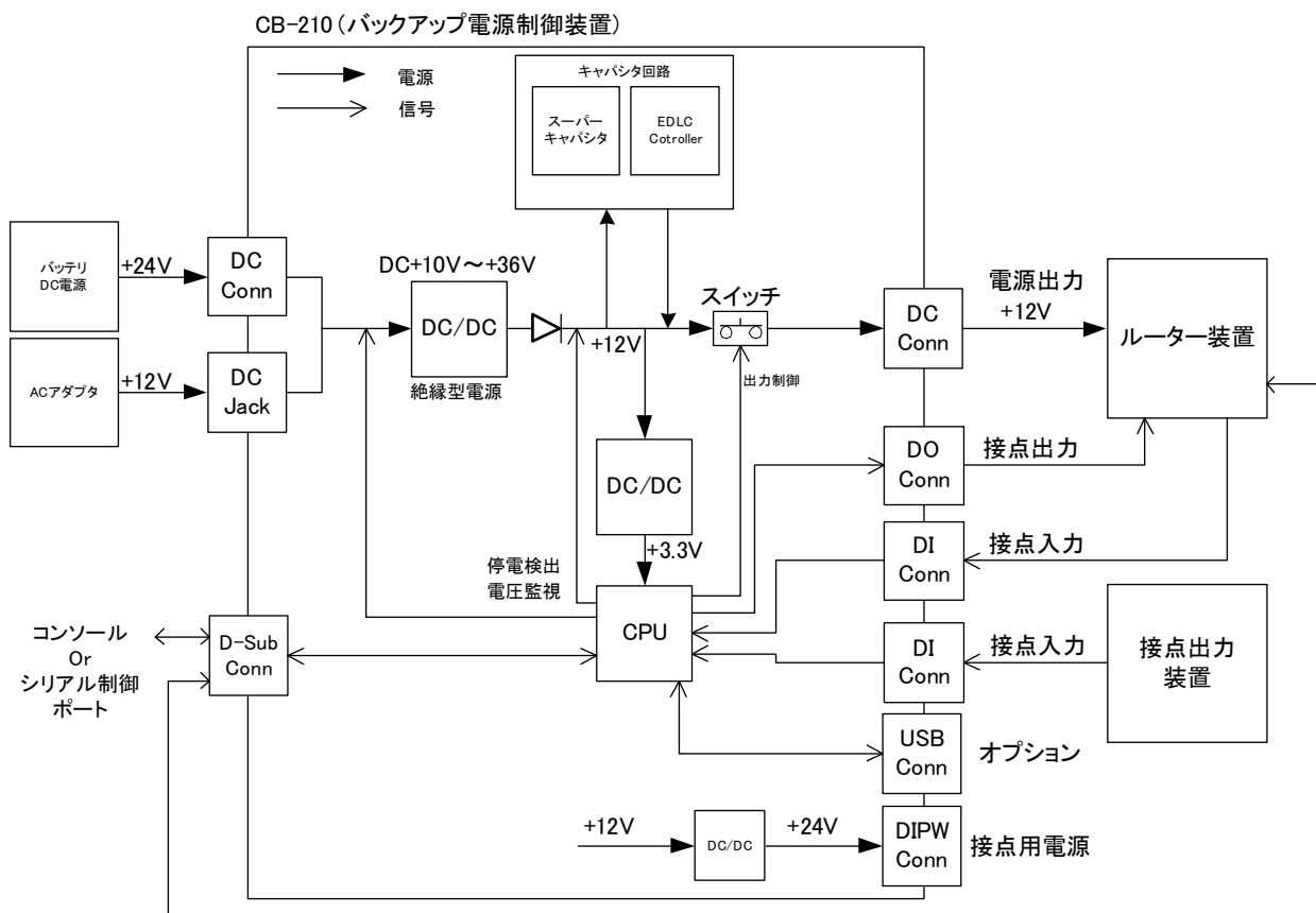
図 3-1 ブロック図
