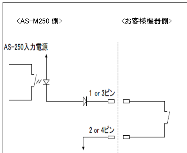
AS-M250 接点入力構成図
