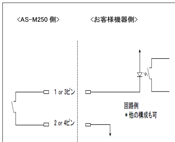
AS-M250 接点出力構成図
