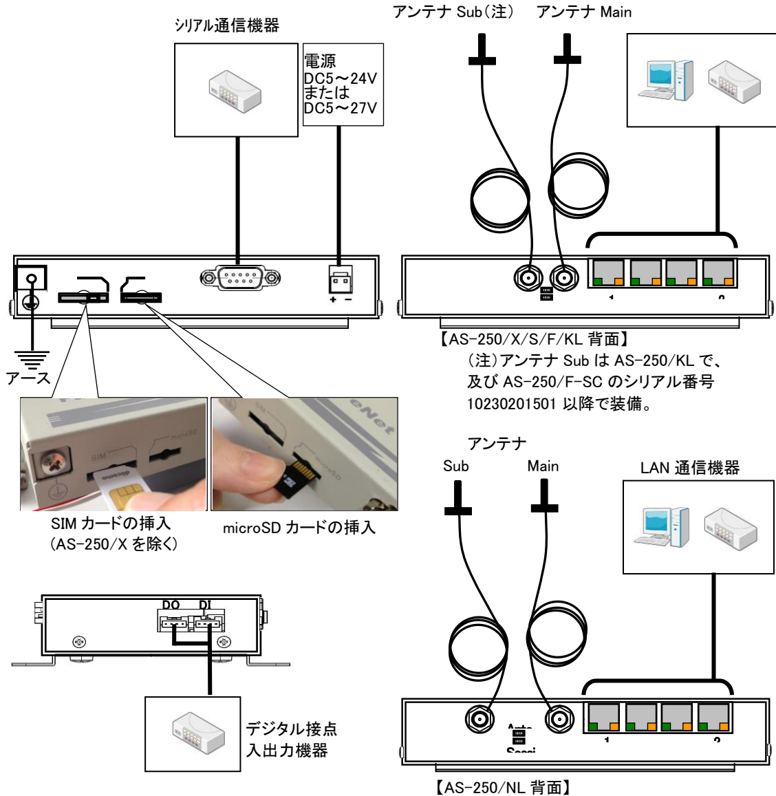
図 2 装置の接続
