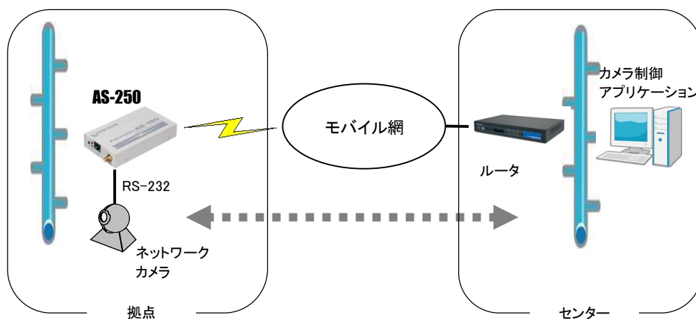
図 4 遠隔地からのカメラ制御
