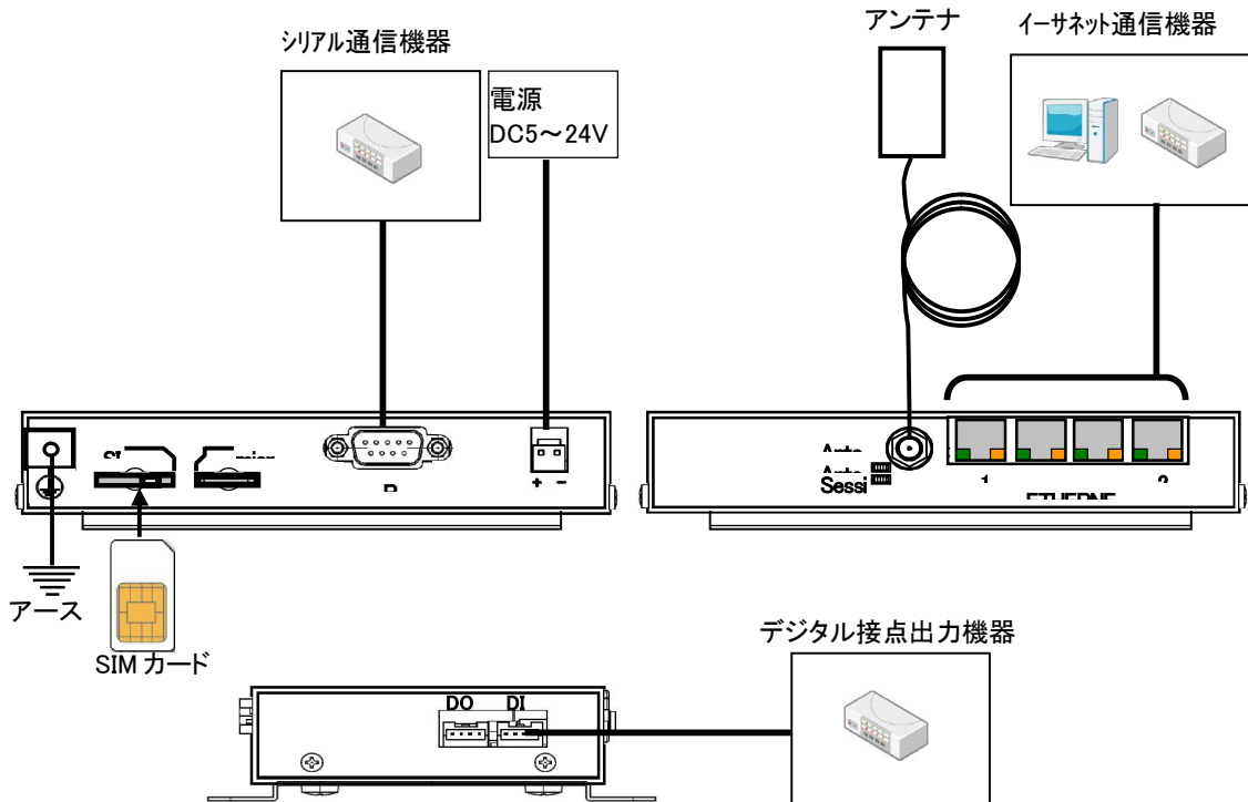
図 2 ケーブルの接続
