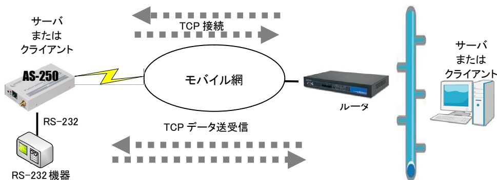
図 7 サーバ&クライアントの利用
