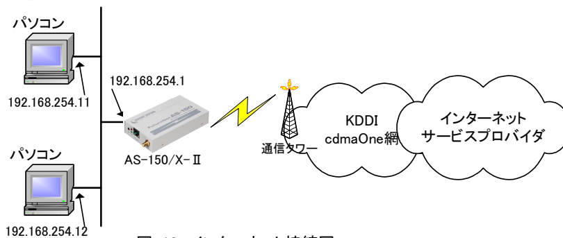
図 10 インターネット接続図
