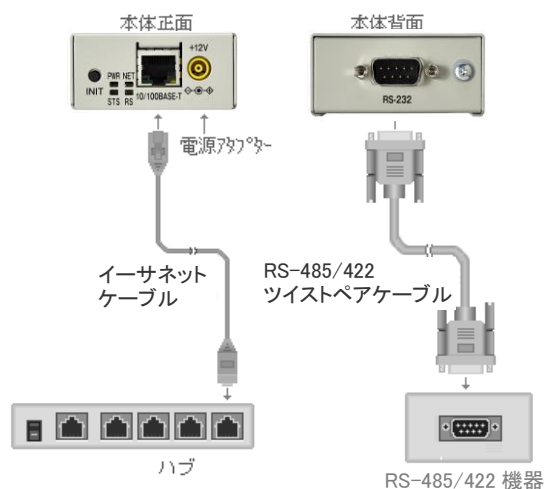
図 3 機器の接続
