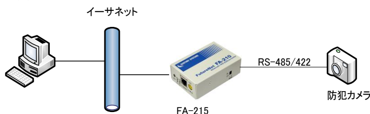
図 1 RS-485/422 装置の接続
