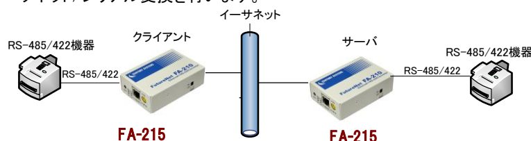
図7 FA-215の対向接続
