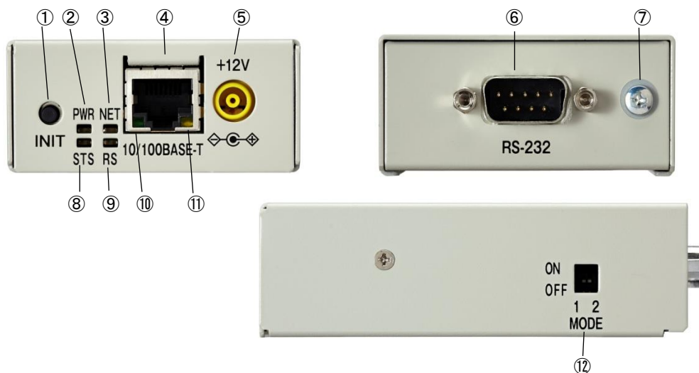
図 2 側面図
