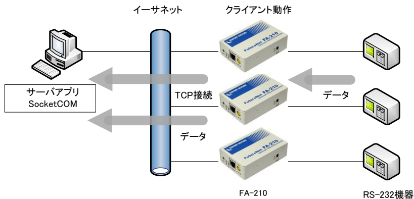
図 7 FA-210 のクライアント機能の利用
