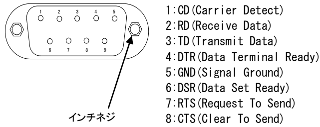
図 4 D-Sub9 ピンコネクタ
