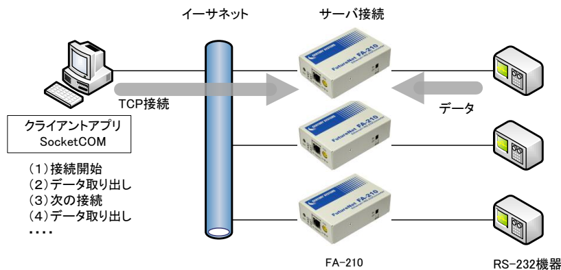
図 6 FA-210 のサーバ機能の利用
