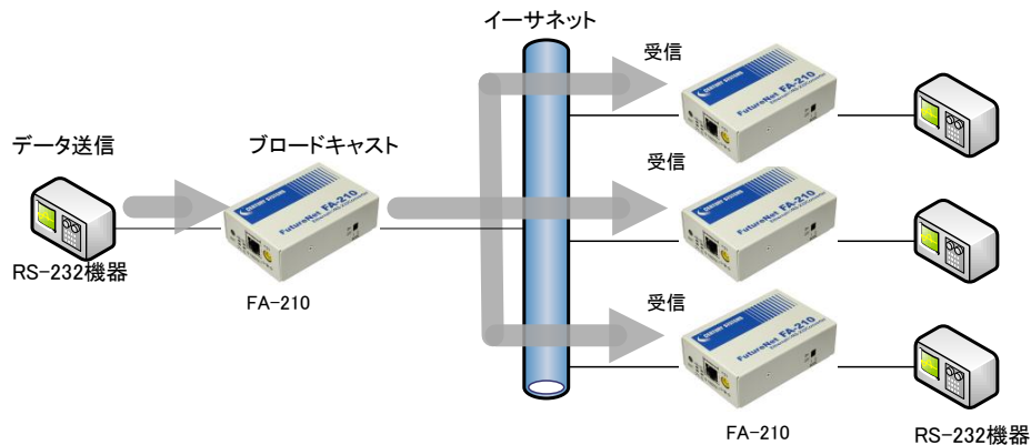
図 11 ブロードキャストによる送信
