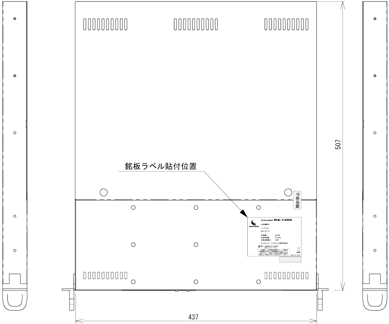
左側面図
