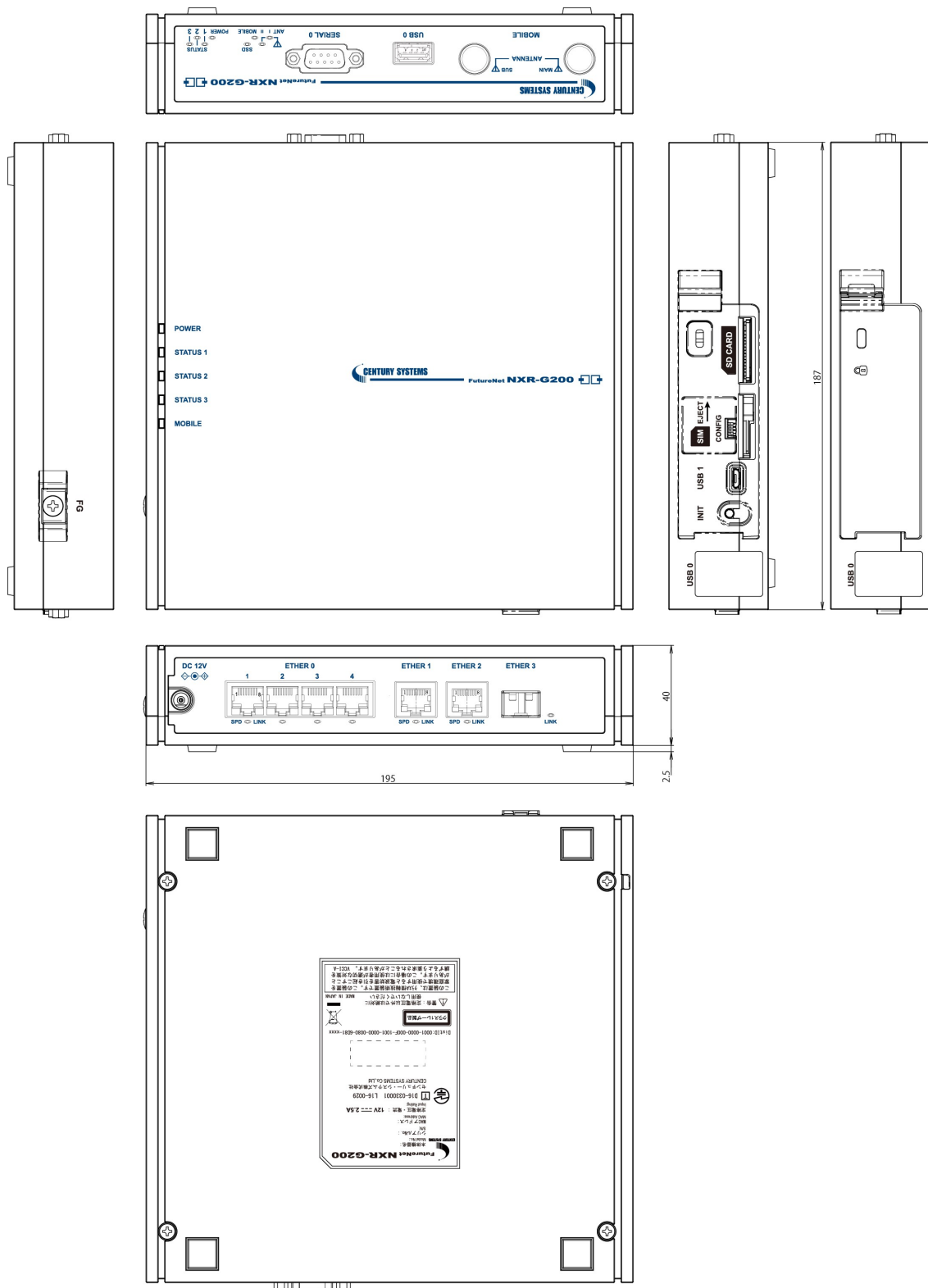
NXR-G240 外觀圖
