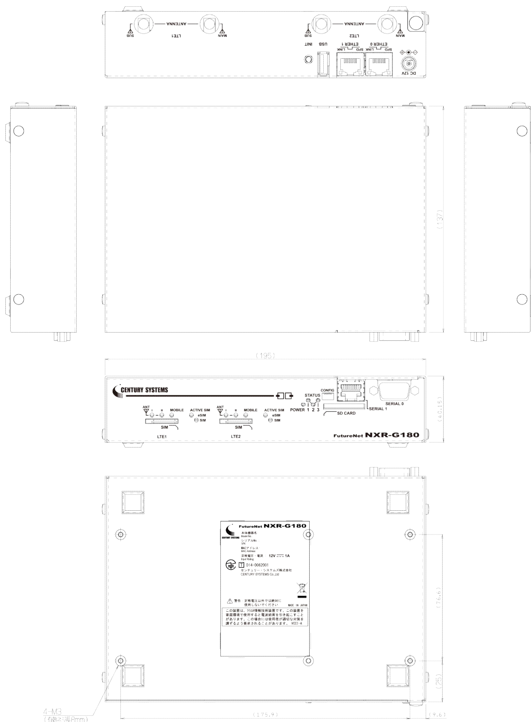
外観図
