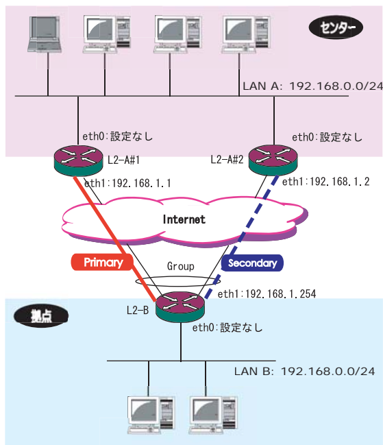
構成図 (例)
