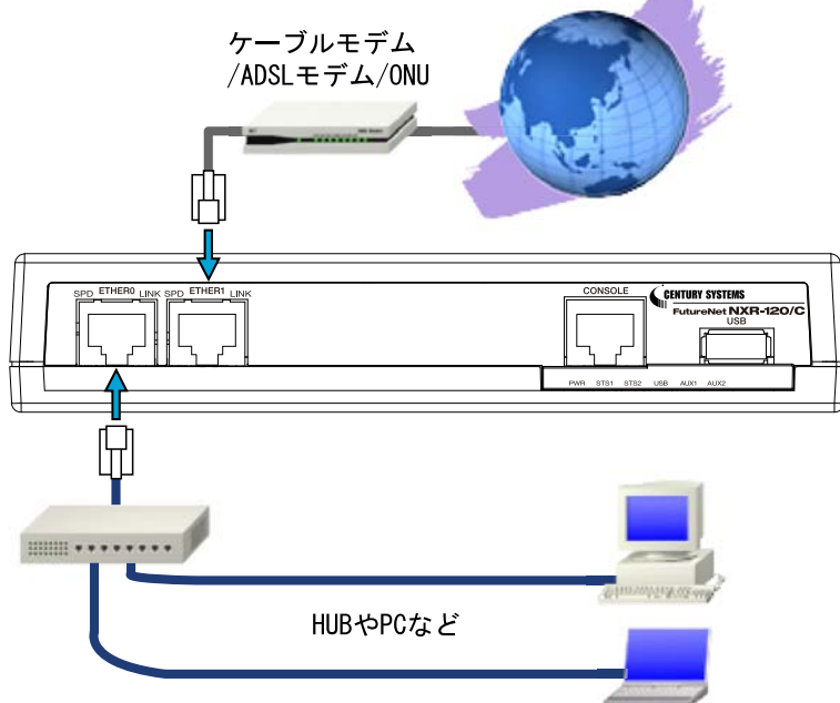
接続図<例> インターネット
