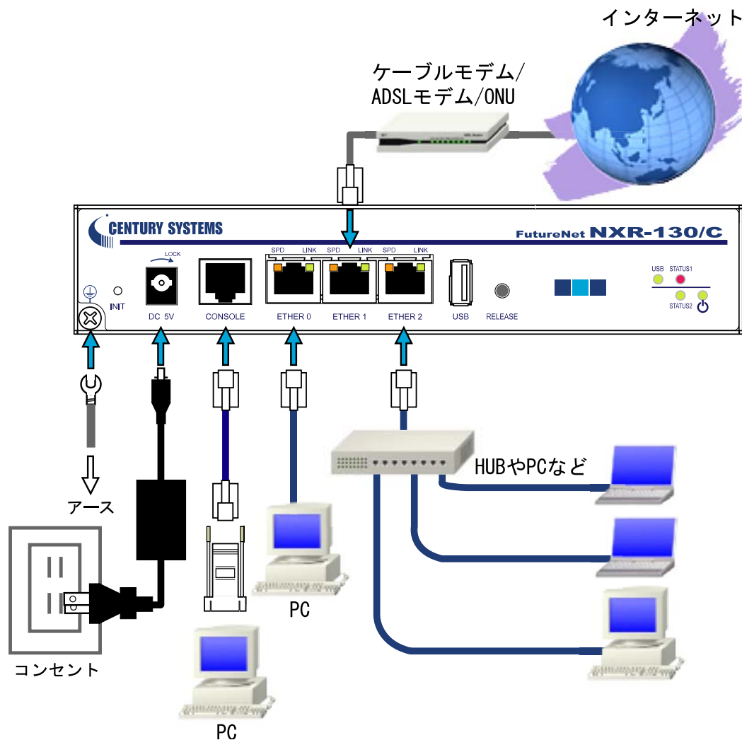
接続図<例>
