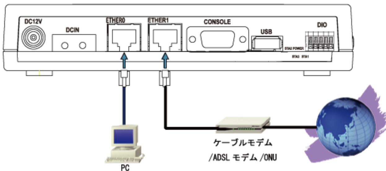
接続図 <例>
