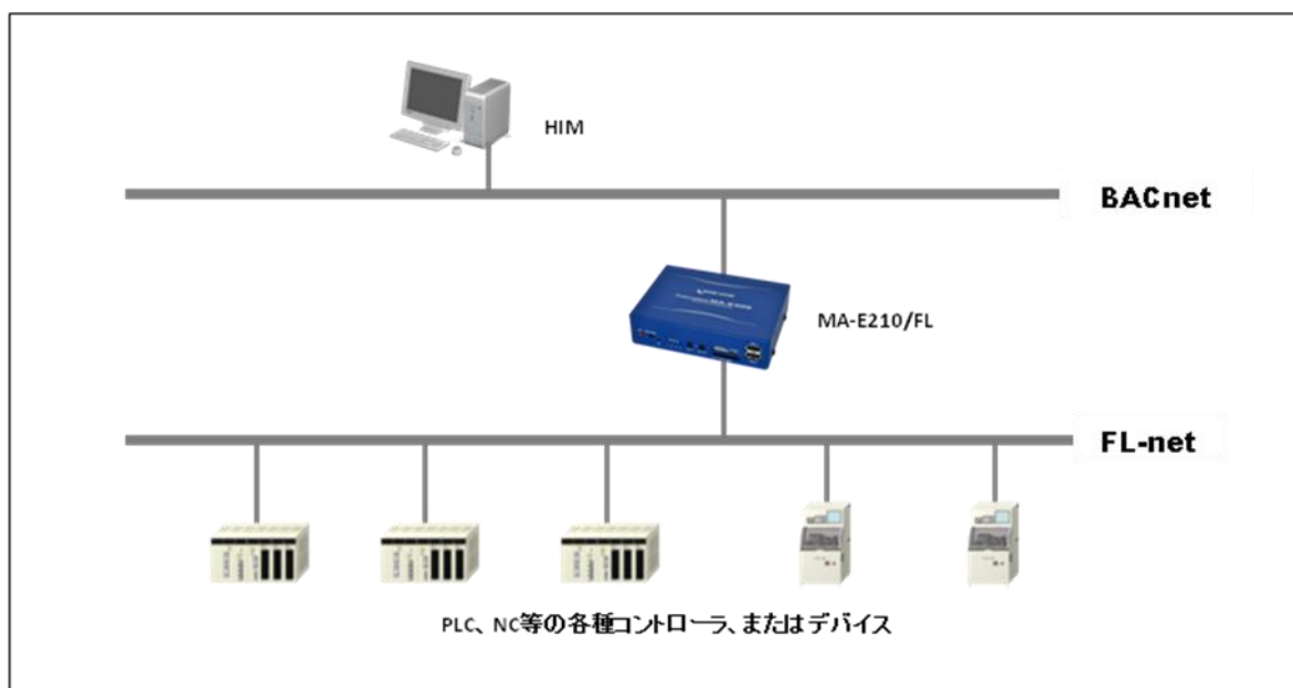
【図：FutureNet MA-E210/FL によるプロトコル変換ゲートウェイの例】
