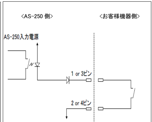
AS-250 接点入力構成図
