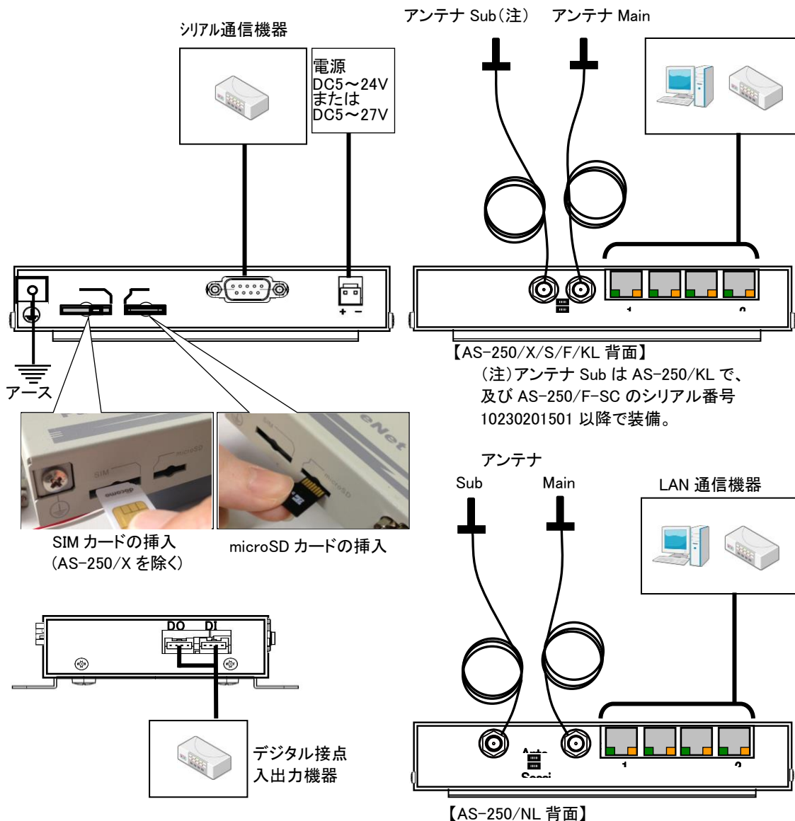
図 2 装置の接続
