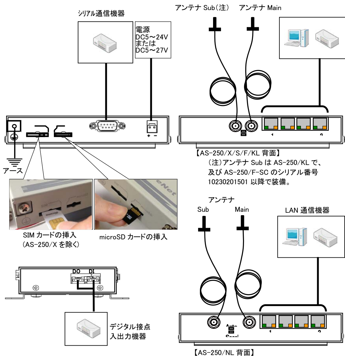
図 2 装置の接続
