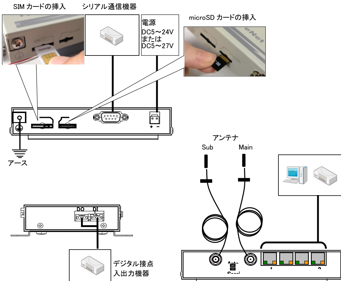
図 2 装置の接続
