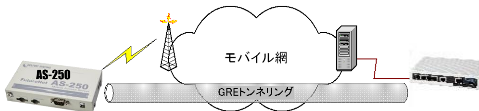
図 3 GRE トンネリングを使う
