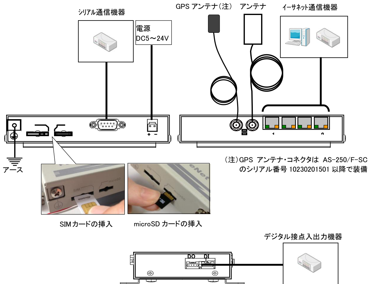
図 2 装置の接続
