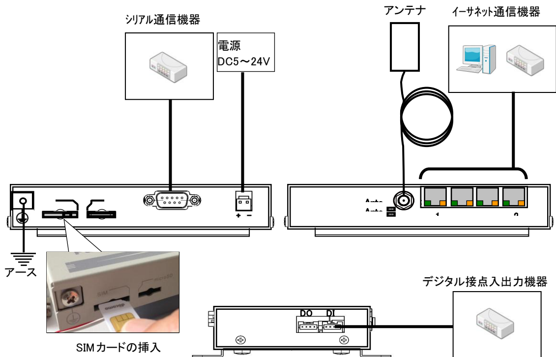
図 2 装置の接続
