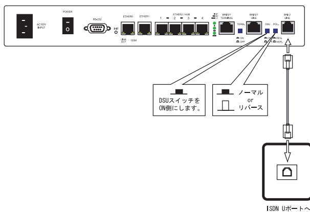
接続図
