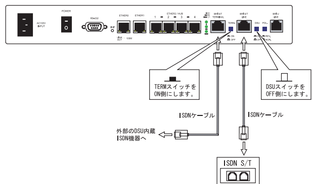
接続図
