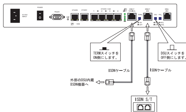
接続図
