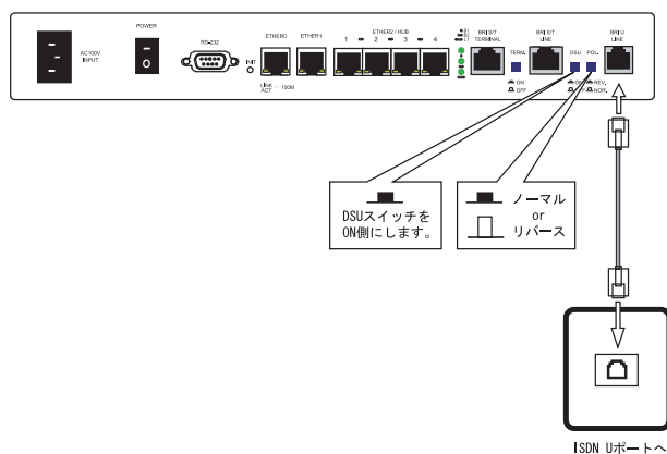
接続図
