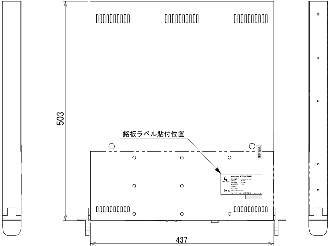
左側面図
