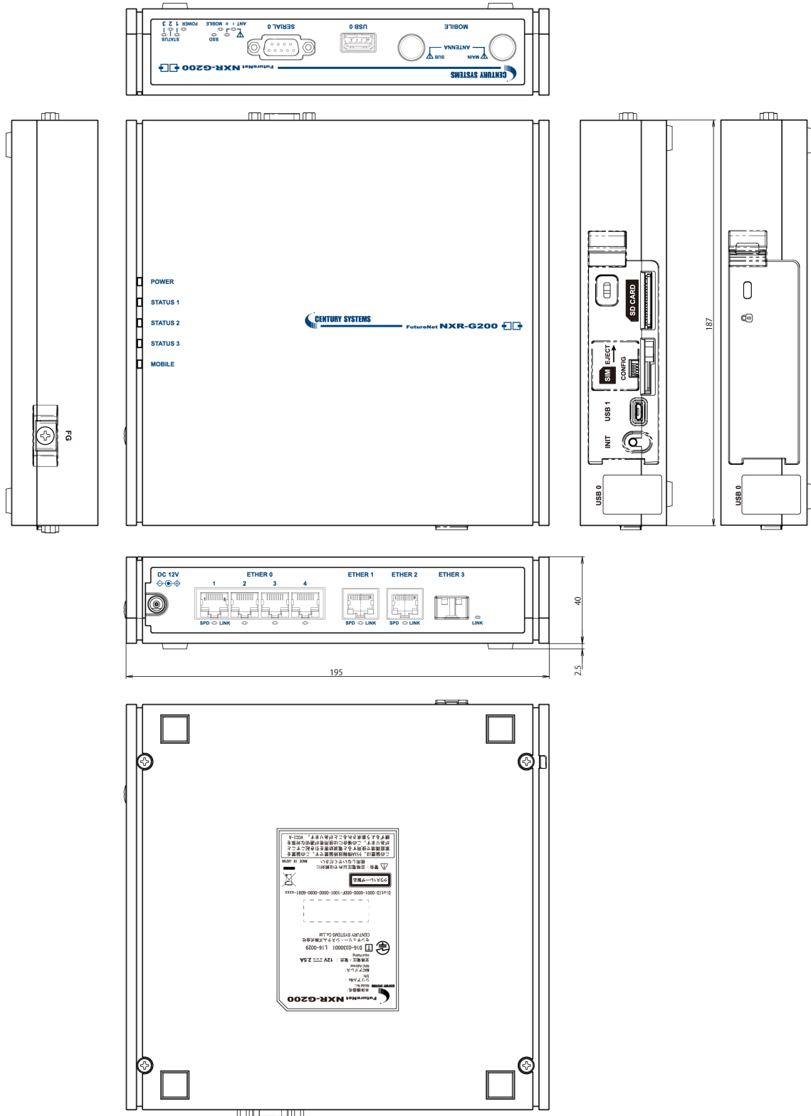
NXR-G240 外觀圖
