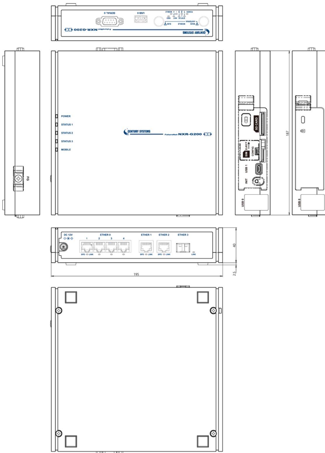
NXR-G240 外観図
