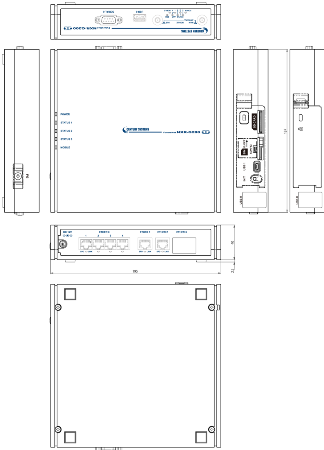
NXR-G240/L 外觀圖
