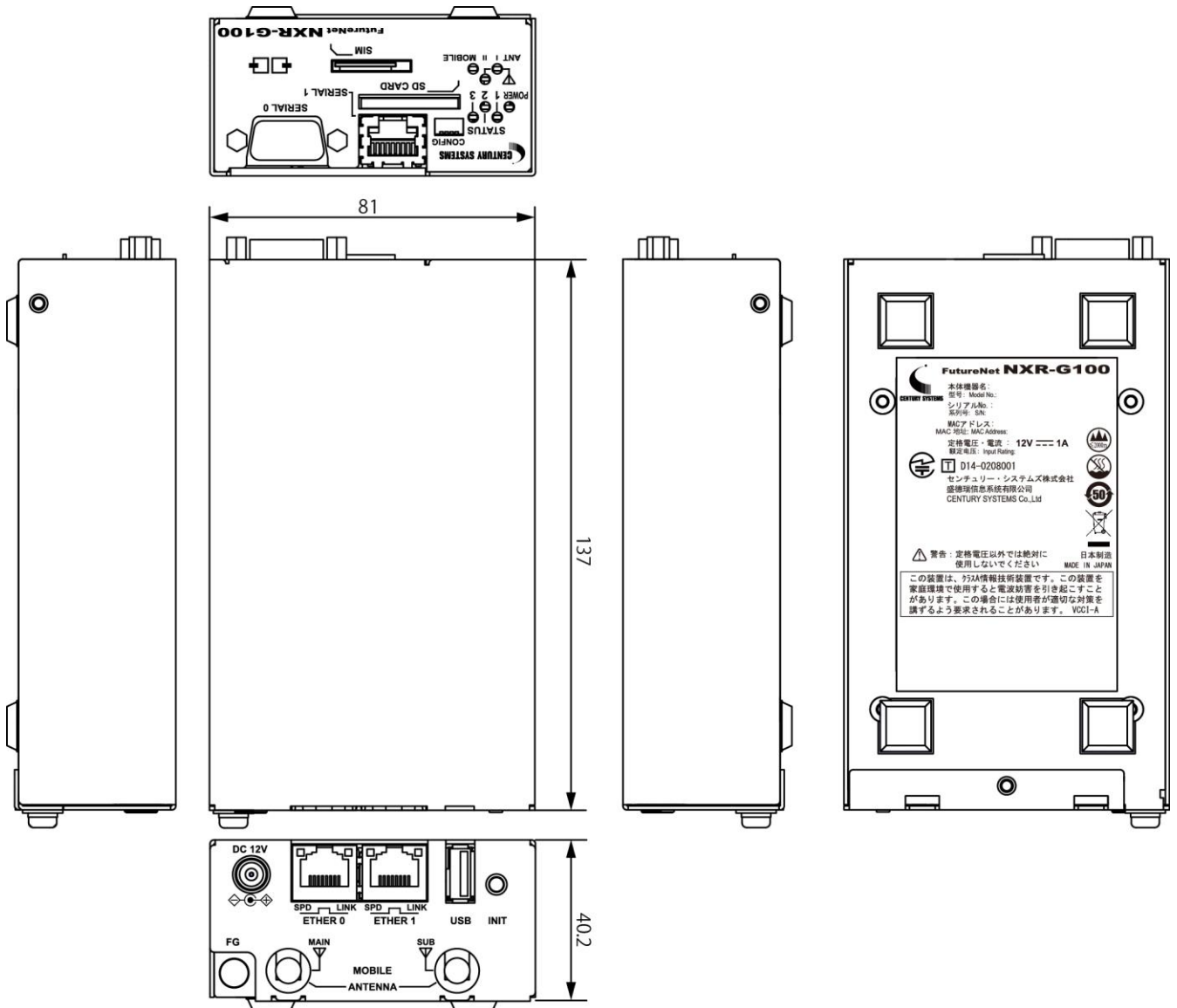
外観図
