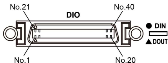
本体側 DIO コネクタ ピン配置
