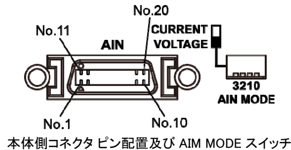
AIN コネクタピン配置表
