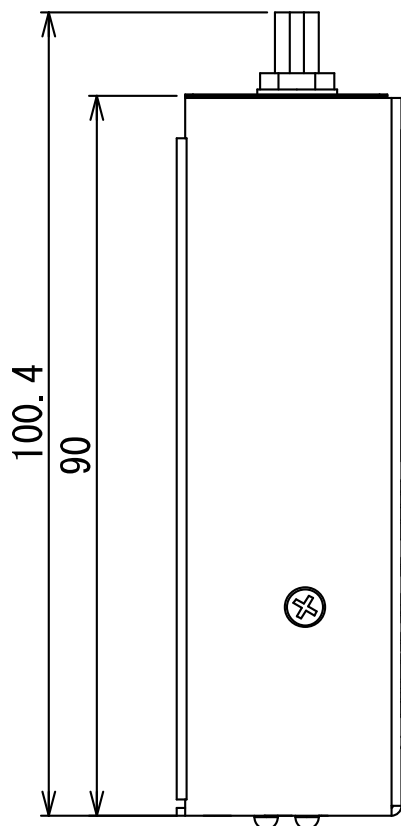
左側面
