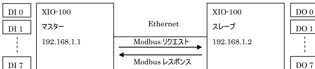
図 8 2 台の XIO-100 を利用した接点延長
