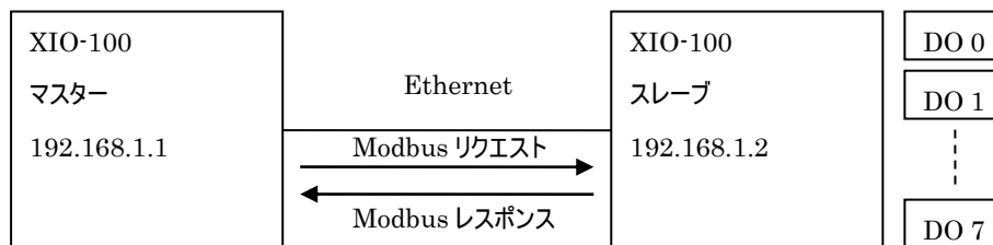
図 7 2 台の XIO-100 を利用した遠隔接点出力
