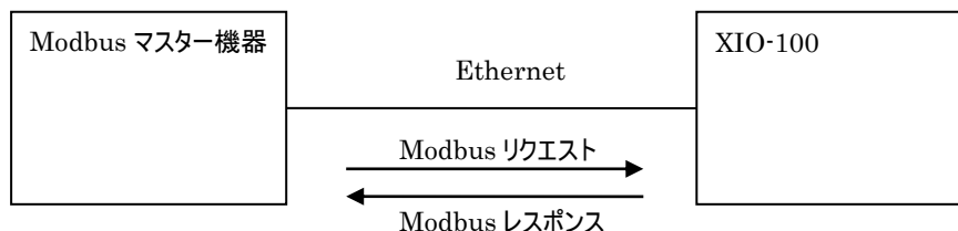
図 6 Modbus マスター機器と Ethernet で接続
