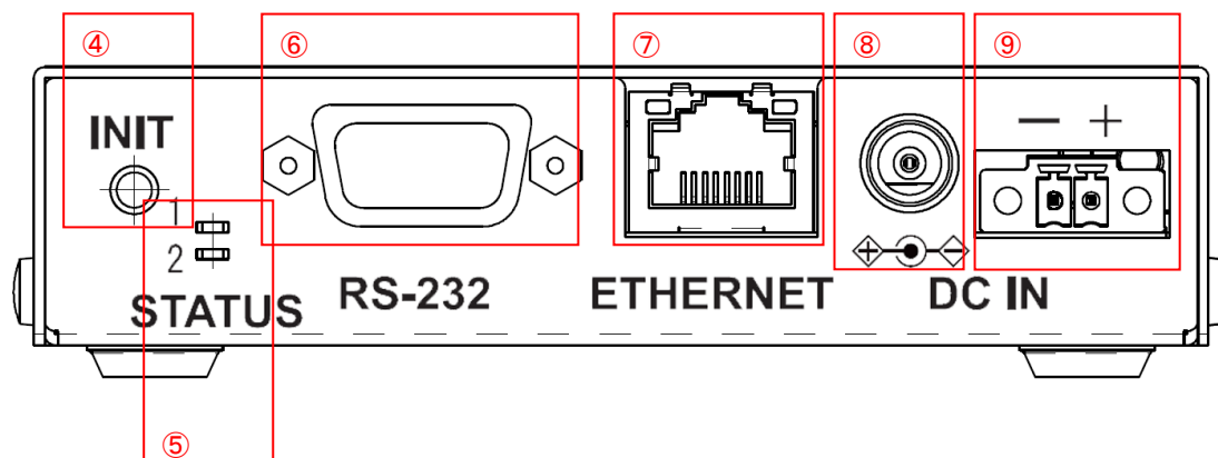
図 2 装置背面図
