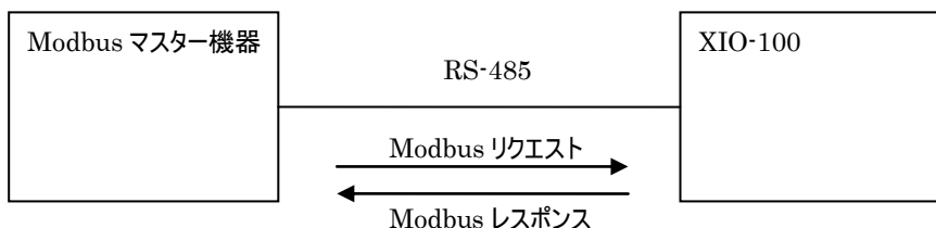
図 4 Modbus マスター機器と RS-485 で接続
