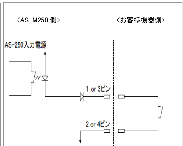
AS-M250 接点入力構成図
