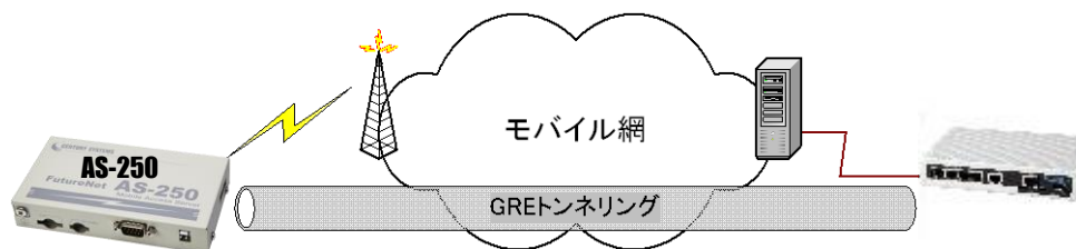
図 2 GRE トンネリングを使う
