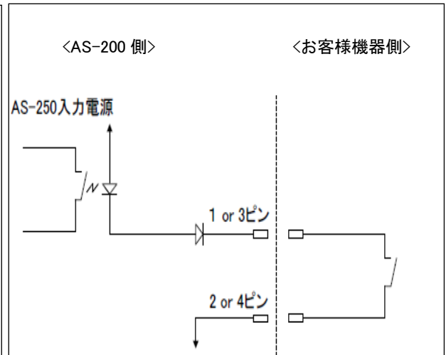
AS-200 接点入力構成図
